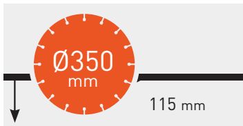
Max. Schnitttiefe
